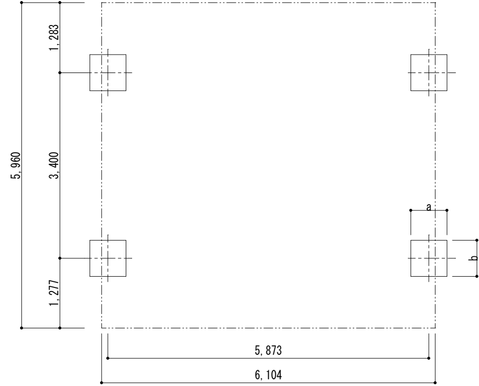
■ 基礎配置図
